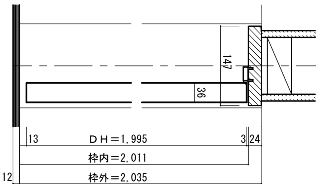
■縦断面図
