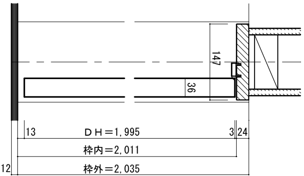
■縦断面図
